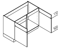
SO Spülenunterschrank ↳ 80/90/100/120 ↓ 75 ↙ 60/50
