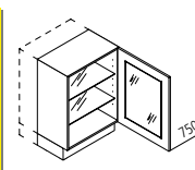
UDDV Unterschrank mit Glasstür (programmabhängig) ↔ 40/45/50/60 ↓ 75/90 ↙ 60/39
