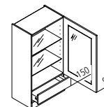
HASKV Aufsatzschrank mit Glasür (programmabhängig) ↳ 45/50/60 ↓ 115 ↶ 35
