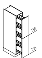
VVA Vorratsschrank ↔ 30/40 ↓ 135/150 ↶ 60
