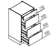
VAK Vorratsschrank ↳ 30/40/45/50/60 ↓ 105 ↶ 60/50
