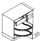
UEA Unterschrank-Ecke ↳ 110/115/125 ↓ 75 ↙ 60
