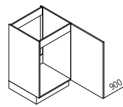
SOD Spülenunterschrank ↔ 45/50/60 ↓ 90 ↙ 60
