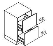
UZ Auszugsschrank ↔ 30/40/45/50/60/80/90/100/120 ↓ 90 ↙ 60/50/39
