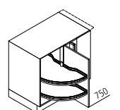
UEAD Unterschrank-Ecke ↳ 110/115/125 ↓ 75 ↙ 60
