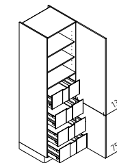
VI Vorratsschrank ↔ 40/45/50/60 ↓ 195/210/225 ↶ 60/50/35
