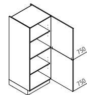
V Vorratsschrank ↔ 30/40/45/50/60 ↓ 135/150 ↶ 60/50/35
