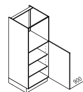
GB Geräteschrank für Backofen oder Mikrowelle ↔ 60 ↓ 135/150 ↶ 60
