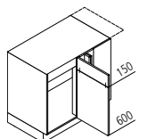
UESA Spülenunterschrank-Ausgleichsecke ↳ 110/115/125 ↓ 75 ↙ 60
