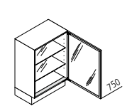
UDDDR Unterschrank mit Glasstür DR ↔ 40/45/50/60 ↓ 75/90 ↙ 39
