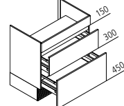
KAK-ML Kochstellenschrank für Muldenlüfter ↔ 60/80/90/100/120 ↓ 75 ↙ 60
