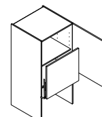
HAL Aufsatzschrank mit Lifttür ↳ 60 ↓ 115/130/145 ↶ 60
