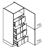
VI Vorratsschrank ↔ 40/45/50/60 ↓ 135/150 ↶ 60/50/35
