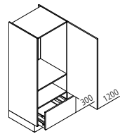
GKA Geräteschrank für Kühlschrank / Nische 880 mm ↔ 60 ↓ 135/150 ↶ 60
