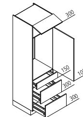
GKAK Geräteschrank für Kühlschrank / Nische 1025 mm ↔ 60 ↓ 195/210/225 ↶ 60
