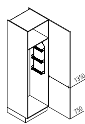
VB Besenschrank ↔ 30/40/45/50/60 ↓ 195/210/225 ↶ 60/50
