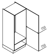
GK Geräteschrank für Kühlschrank / Nische 1225 mm ↔ 60 ↓ 135/150 ↶ 60
