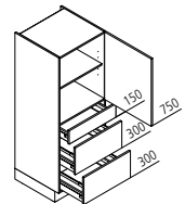
VAK Vorratsschrank ↔ 30/40/45/50/60 ↓ 135/150 ↶ 60/50
