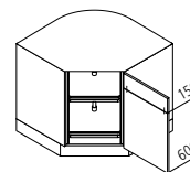
UET Unterschrank-Ecke ↳ 90 ↓ 75 ↙ 60
