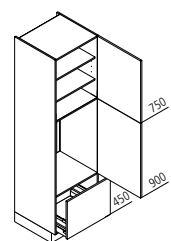
GKA Geräteschrank für Kühlschrank / Nische 880 mm ↔ 60 ↓ 195/210/225 ↶ 60
