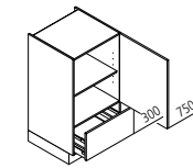
VA Vorratsschrank ↳ 30/40/45/50/60 ↓ 105 ↶ 60/50
