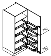
VVK Vorratsschrank ↔ 60 ↓ 135/150 ↶ 60
