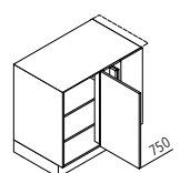
UEEAD Unterschrank-Ecke ↳ 110/115/125 ↓ 75 ↙ 60/50
