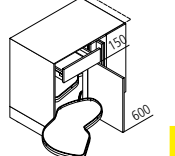
UELA Unterschrank-Ecke ↳ 110/115/125 ↓ 75 ↙ 60
