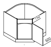
UES Spülenunterschrank-Ecke ↳ 90 ↓ 75 ↙ 60
