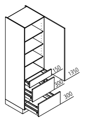
VAK Vorratsschrank ↔ 30/40/45/50/60 ↓ 195/210/225 ↶ 60/50
