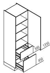
VZ Vorratsschrank ↔ 30/40/45/50/60 ↓ 195/210/225 ↶ 60/50
