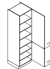
V Vorratsschrank ↔ 30/40/45/50/60 ↓ 195/210/225 ↶ 60/50/35
