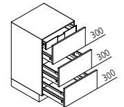
UAZI Auszugsschrank ↔ 30/40/45/50/60/80/90/100/120 ↓ 90 ↙ 60/50/39
