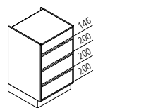
URI Unterschrank-Regal mit Schubkästen ↔ 60/90 ↓ 90 ↙ 60/39
