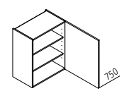
H Hängeschrank
