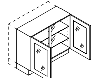
UDDV Unterschrank mit Glasstür (programmabhängig) ↔ 80/90/100/120 ↓ 75/90 ↙ 60/39
