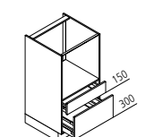
GBAS Geräteschrank für Backofen oder Mikrowelle ↳ 60 ↓ 105 ↶ 60
