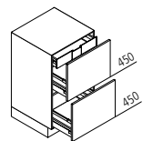
UZI Auszugsschrank ↔ 30/40/45/50/60/80/90/100/120 ↓ 90 ↙ 60/50/39
