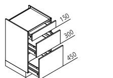
KUAK Kochstellenschrank ↔ 60/80/90/100/120 ↓ 90 ↙ 60
