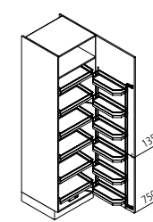
VVK Vorratsschrank ↔ 60 ↓ 195/210/225 ↶ 60
