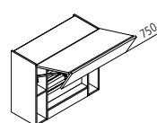
HWUFK Faltklappenschrank für integrierte Abzughaube
