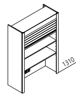
H AJ Aufsatzschrank mit Jalousie in Metall-Optik ↳ 50/60/80/90 ↓ 115/130/145 ↶ 35/50/60
