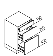
UAK Auszugsschrank ↔ 30/40/45/50/60/80/90/100/120 ↓ 90 ↙ 60/50/39
