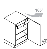
UDDI Unterschrank ↔ 40/45/50/60 ↓ 90 ↙ 60/50
