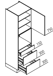
GBAK Geräteschrank für Backofen / Mikrowelle ↔ 60 ↓ 195/210/225 ↶ 60
