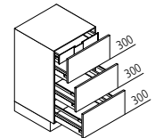
UAZI Auszugsschrank ↔ 30/40/45/50/60/80/90/100/120 ↓ 90 ↙ 60/50/39
