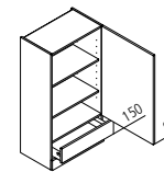
HASK Aufsatzschrank ↳ 45/50/60 ↓ 115/ ↶ 35
