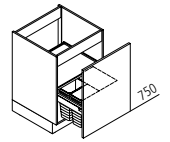
SABHD Spülenunterschrank mit hängendem Abfalltrennsystem
