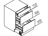
UAKS Auszugsschrank mit Großraumauszug ↔ 60/80/90/100 ↓ 75 ↙ 60
