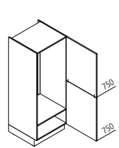
GK Geräteschrank für Kühlschrank / Nische 1225 mm ↔ 60 ↓ 135/150 ↶ 60
