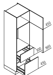
GKZ Geräteschrank für Kühlschrank / Nische 880 mm ↔ 60 ↓ 195/210/225 ↶ 60
