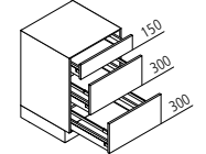
UAK Auszugsschrank ↔ 30/40/45/50/60/80/90/100/120 ↓ 75 ↙ 60/50/75/39
