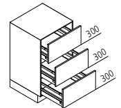
UAZ Auszugsschrank ↔ 30/40/45/50/60/80/90/100/120 ↓ 90 ↙ 60/50/39
