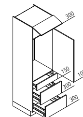
GKAK Geräteschrank für Kühlschrank / Nische 1025 mm ↔ 60 ↓ 195/210/225 ↶ 60
