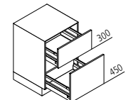
UZ Auszugsschrank ↔ 30/40/45/50/60/80/90/100/120 ↓ 75 ↙ 60/50/75/39
