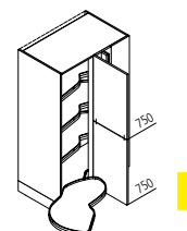
VECLA Vorratsschrank- Ecke ↔ 110/115/125 ↓ 135/150 ↶ 60
