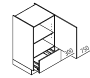
VA Vorratsschrank ↳ 30/40/45/50/60 ↓ 105 ↶ 60/50
