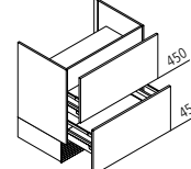
KUZ Kochstellenschrank für Muldenlüfter ↔ 60/80/90/100/120 ↓ 75 ↙ 60
