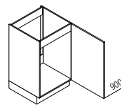
SOD Spülenunterschrank ↔ 45/50/60 ↓ 90 ↙ 60
