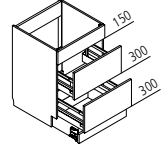
SABSD Spülenunterschrank mit Großraum-Sockelauszug
