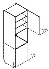
GSSB Geräteschrankbau für Geschirrspüler / Backofen ↔ 60 ↓ 195/210/225 ↶ 60
