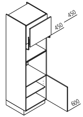
GBL Geräteschrank mit Lifttür für Backofen / Mikrowelle ↔ 60 ↓ 195/210/225 ↶ 60
