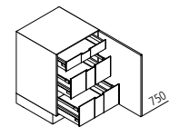
UIDD Unterschrank ↔ 40/45/50/60 ↓ 75 ↙ 60/50/39
