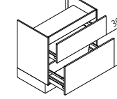
KUZ Kochstellenschrank für Muldenlüfter
