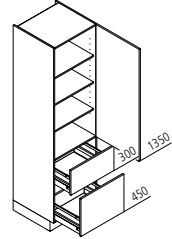
VZ Vorratsschrank ↔ 30/40/45/50/60 ↓ 195/210/225 ↶ 60/50
