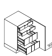
UIDD Unterschrank ↔ 40/45/50/60 ↓ 90 ↙ 60/50/39
