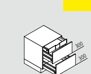
UAZI Auszugsschrank ↔ 30/40/45/50/60/80/90/100 ↓ 60 ↙ 60/50
