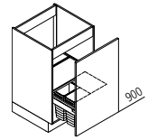
SABHD Spülenunterschrank mit Abfalltrennsystem ↔ 45/50/60 ↓ 90 ↙ 60
