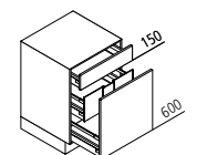
UATIA Auszugsschrank ↔ 30/40/45/50/60/80/90/100/120 ↓ 75 ↙ 60/50
