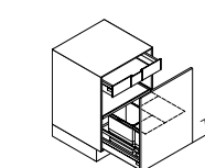
UABDG Auszugsschrank mit Abfalleimer ↔ 40/45/50/60 ↓ 75 ↙ 60
