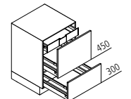
UAZI Auszugsschrank ↔ 30/40/45/50/60/80/90/100/120 ↓ 75 ↙ 60/50
