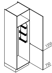
VB Besenschrank ↔ 30/40/45/50/60 ↓ 195/210/225 ↶ 60/50
