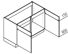
SO Spülenunterschrank
