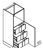
GBI Geräteschrank für Backofen oder Mikrowelle ↔ 60 ↓ 135/150 ↶ 60
