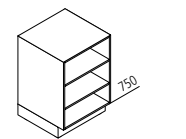
UR Unterschrank-Regal ↔ 15/20/25/30/35/40/45/50/55/60 ↓ 75 ↙ 60/39
