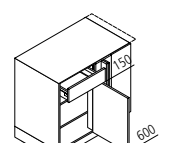
UEEA Unterschrank-Ecke
