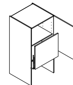
HAL Aufsatzschrank mit Lifttür ↳ 60 ↓ 115/130/145 ↶ 60
