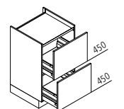
KUZ Kochstellenschrank ↔ 60/80/90/100/120 ↓ 90 ↙ 60
