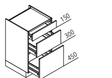
KUAK Kochstellenschrank ↔ 60/80/90/100/120 ↓ 90 ↙ 60
