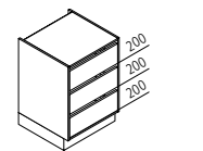
URI Unterschrank-Regal mit Schubkästen ↔ 60/90 ↓ 75 ↙ 60
