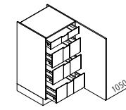
VI Vorratsschrank ↳ 40/45/50/60 ↓ 105 ↶ 60/50/35
