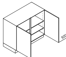
UDD Unterschrank ↔ 80/90/100/120 ↓ 90 ↙ 60/50/39
