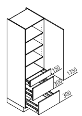
VAK Vorratsschrank ↔ 30/40/45/50/60 ↓ 195/210/225 ↶ 60/50
