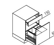
UABG Auszugsschrank mit Abfalleimer ↔ 40/45/50/60 ↓ 75 ↙ 60
