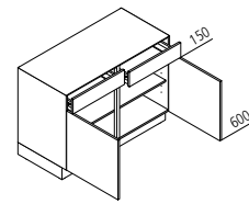
U Unterschrank ↔ 80/90/100/120 ↓ 75 ↙ 60/50/39
