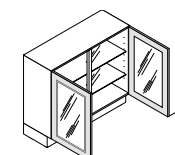
UDDDN Unterschrank mit Glasstür DN ↔ 80/90/100/120 ↓ 75/90 ↙ 39
