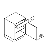
U Unterschrank ↔ 30/40/45/50/60 ↓ 75 ↙ 60/50/39
