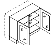
UDDV Unterschrank mit Glasstür (programmabhängig) ↔ 80/90/100/120 ↓ 75/90 ↙ 60/39
