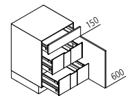
UI Unterschrank ↔ 40/45/50/60 ↓ 75 ↙ 60/50/39
