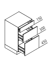
UAK Auszugsschrank ↔ 30/40/45/50/60/80/90/100/120 ↓ 90 ↙ 60/50/39
