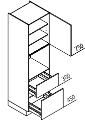
GBZ Geräteschrank für Backofen / Mikrowelle ↔ 60 ↓ 195/210/225 ↶ 60
