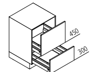
UAZ Auszugsschrank ↔ 30/40/45/50/60/80/90/100/120 ↓ 75 ↙ 60/50
