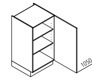
V Vorratsschrank ↳ 30/40/45/50/60 ↓ 105 ↶ 60/50/35
