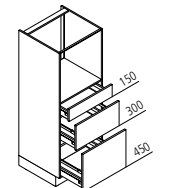
GBZ Geräteschrank für Backofen oder Mikrowelle ↔ 60 ↓ 135/150 ↶ 60
