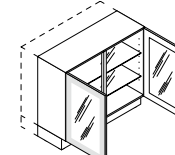
UDDDS Unterschrank mit Glasstür DS ↔ 80/90/100/120 ↓ 75/90 ↙ 60/39
