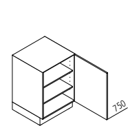
UDD Unterschrank ↔ 30/35/40/45/50/60 ↓ 75 ↙ 60/50/39
