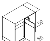
UESA Spülenunterschrank-Ausgleichsecke
