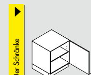
UDD Unterschrank ↔ 30/35/40/45/50/60 ↓ 60 ↙ 60/50/39
