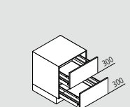
UAZ Auszugsschrank ↔ 30/40/45/50/60/80/90/100/120 ↓ 60 ↙ 60/50
