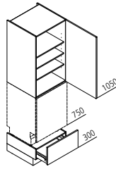
GSSA Geräteschrankbau für Geschirrspüler ↔ 60 ↓ 195/210/225 ↶ 60
